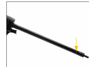
Нанесите несколько капель масла в отверстие трубки затворного механизма
